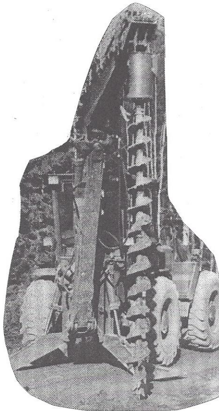
Minborr manövrerad och driven av traktor. Borrens längd cirka 3 meter
