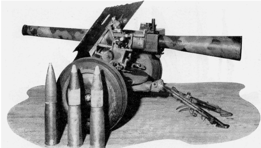
Infanterikanon 10,5 cm m/45.
