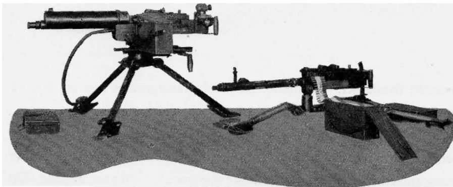
Kulsprutor: till vänster ml'36, till höger m f 42.
