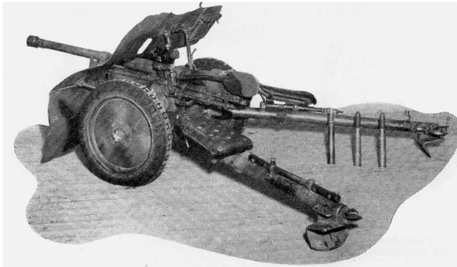
Pansvärnskanon 37 mm m/38.
